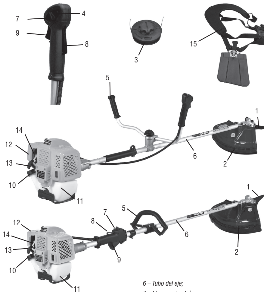
Figura 1 – Componentes
