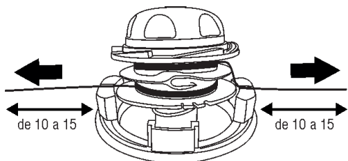
Figura 18 – Comprimento do fio de nylon
