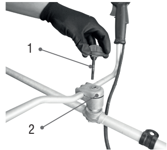
Figura 5 – Montaje final de la manija
