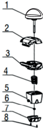
Figura 3 – Componentes del sistema de fijación de la manija
