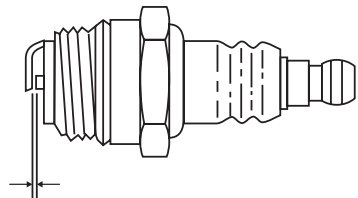
Figura 29 – Distancia de los electrodos de la bujía
