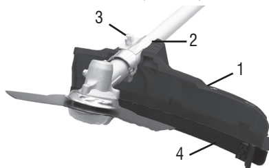
Figura 7 – Montaje de la protección
