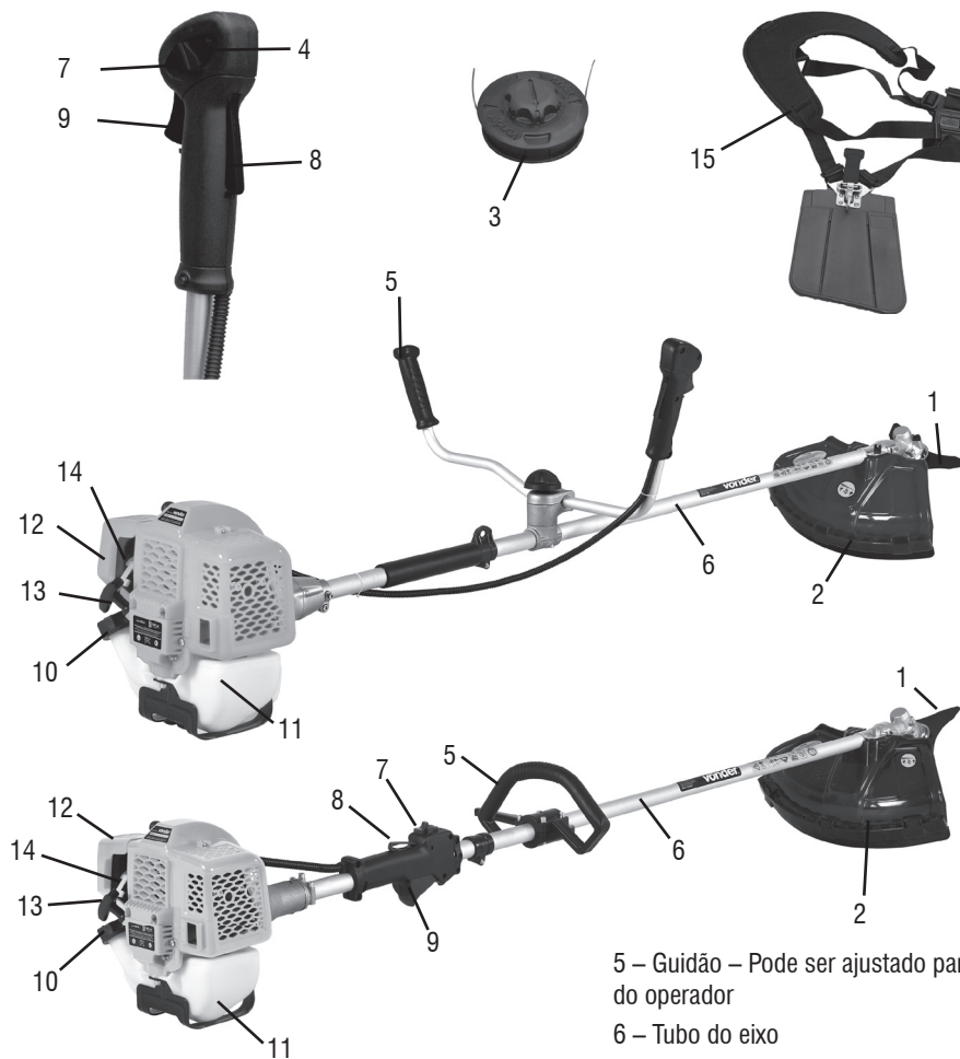
Figura 1 – Componentes
