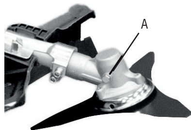
Figura 31 – Lubrificação da caixa de transmissão
