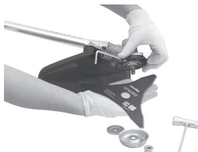
Figura 10 – Posicionando a lâmina
