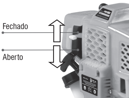
Figura 23 – Afogador
