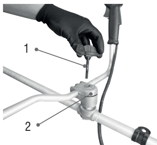
Figura 5 – Montagem final do guidão
