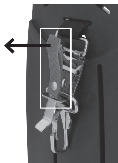
Figura 25 – Sistema de retirada de la desmalezadora del cinto
