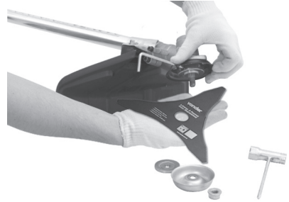
Figura 10 – Posicionando la lámina
