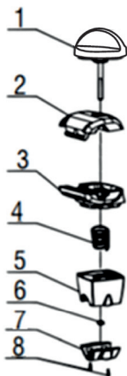
Figura 3 – Componentes do sistema de fixação do guidão
