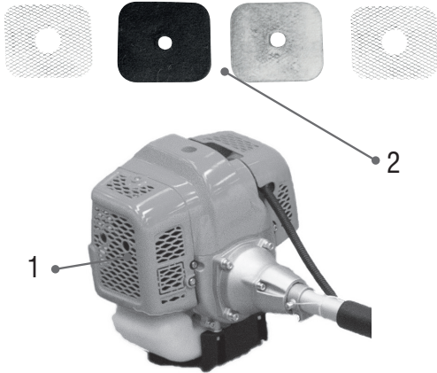
Figura 29 – Elemento filtrante
