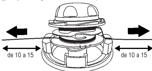
Figura 18 – Largo del hilo de nylon
