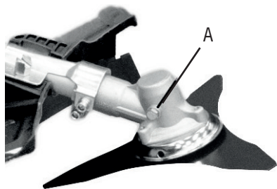
Figura 30 – Lubricación de la caja de transmisión
